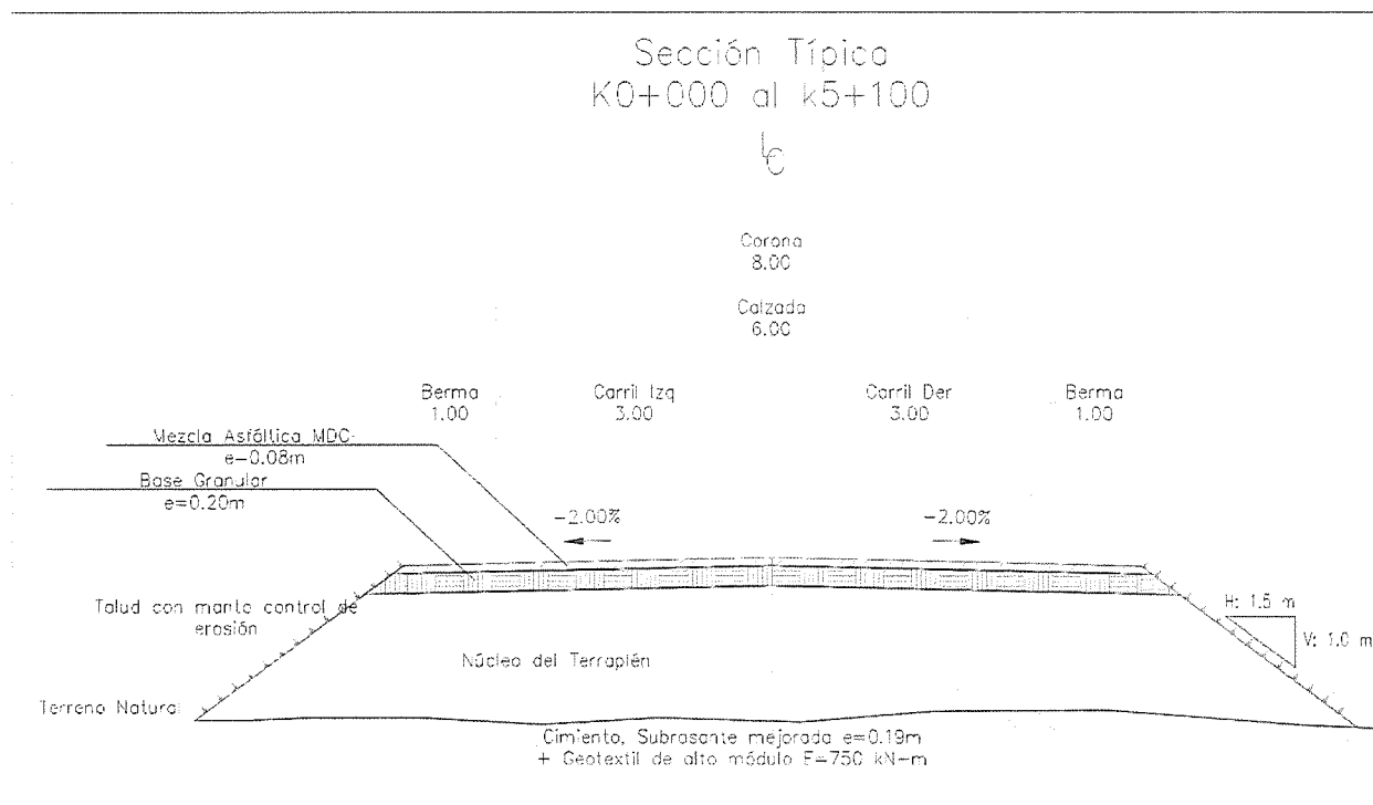
Ilustración 1 Detalle Sección Transversal de la estructura a conformar Fuente: Archivos del proyecto – Diseño Geométrico del Proyecto
